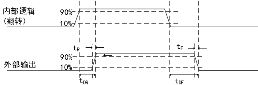
图3-22 光耦输出信号延迟示意
