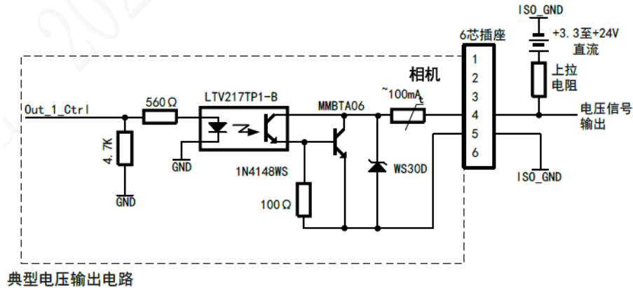
图3-21 Line o 内部电路
