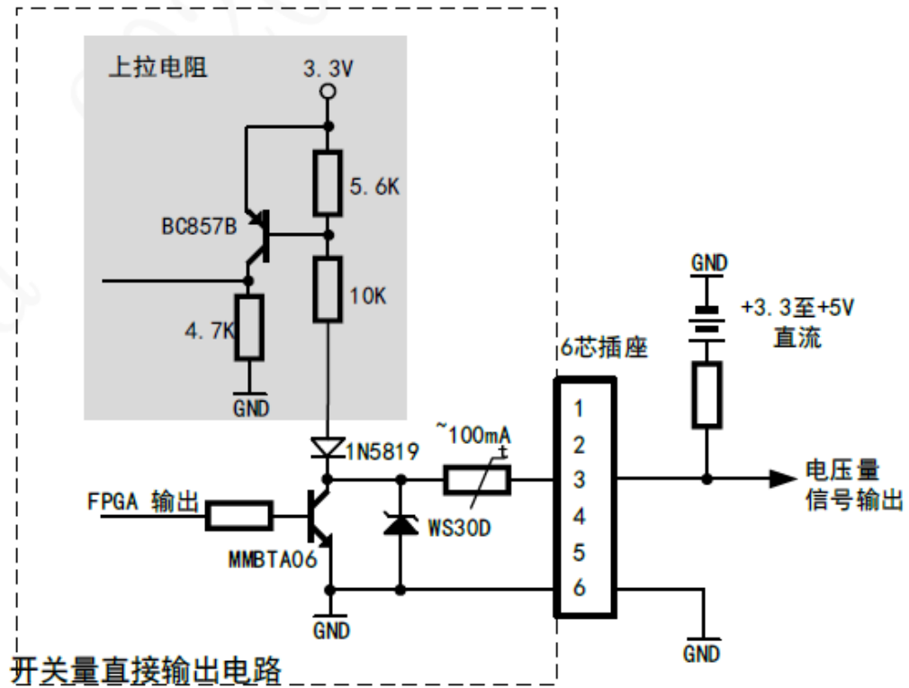
图3-19 GPIO 输出
